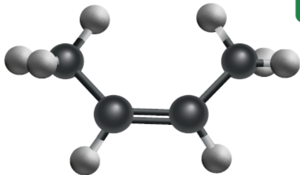
cis - 2 - Buteno
