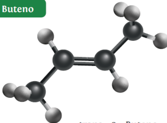
trans - 2 - Buteno
